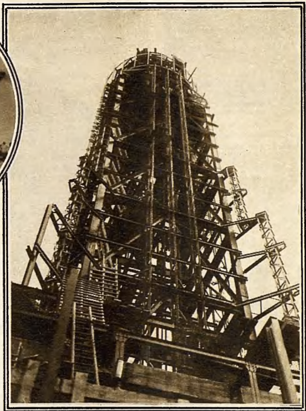
El esqueleto de acero de la torre del edificio Empire State, en Nueva York, donde a media milla de distancia del pavimento se erigirá un mástil para el supuesto anclaje de dirigibles trasatlánticos, en el corazón mismo de la ciudad.
