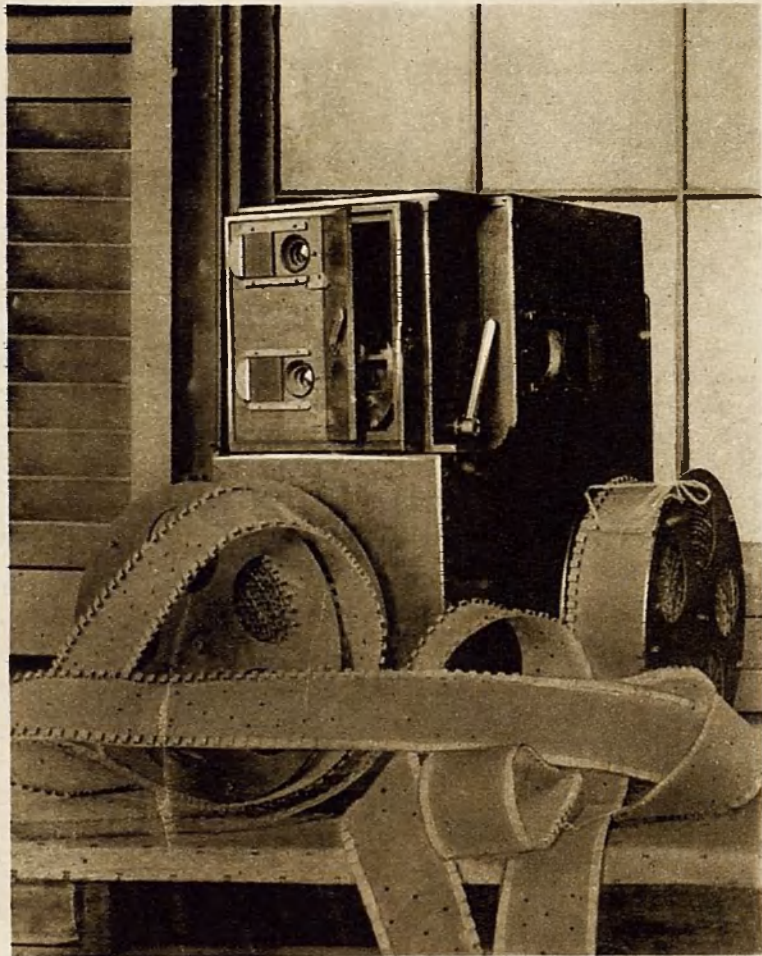
La cámara-proyector de un solo lente que Le Prince construyó en su taller de 160 Woodhouse Lane, en Leeds, Inglaterra, el año de 1888, y con la cual obtuvo fotografías tanto en ese país como en Francia.
