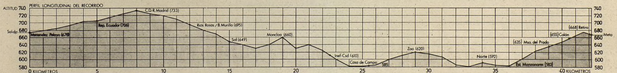
Arriba, plano de la carrera. Abajo, perfil longitudinal
