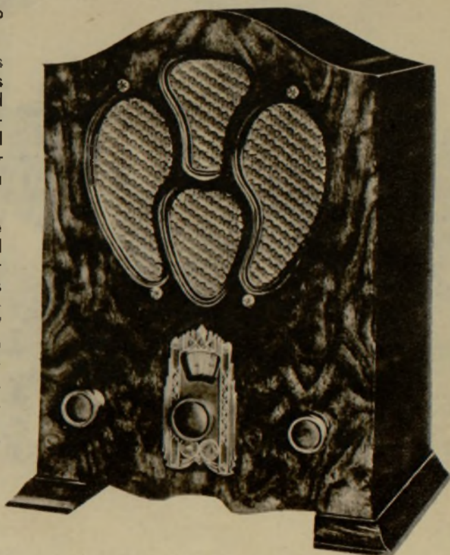
● Modelo R-150 de 4 válvulas, una Pentode. Altavoz dinámico de bobina móvil. Precio: Ptas. 650 para (c. a.) Ptas. 650
