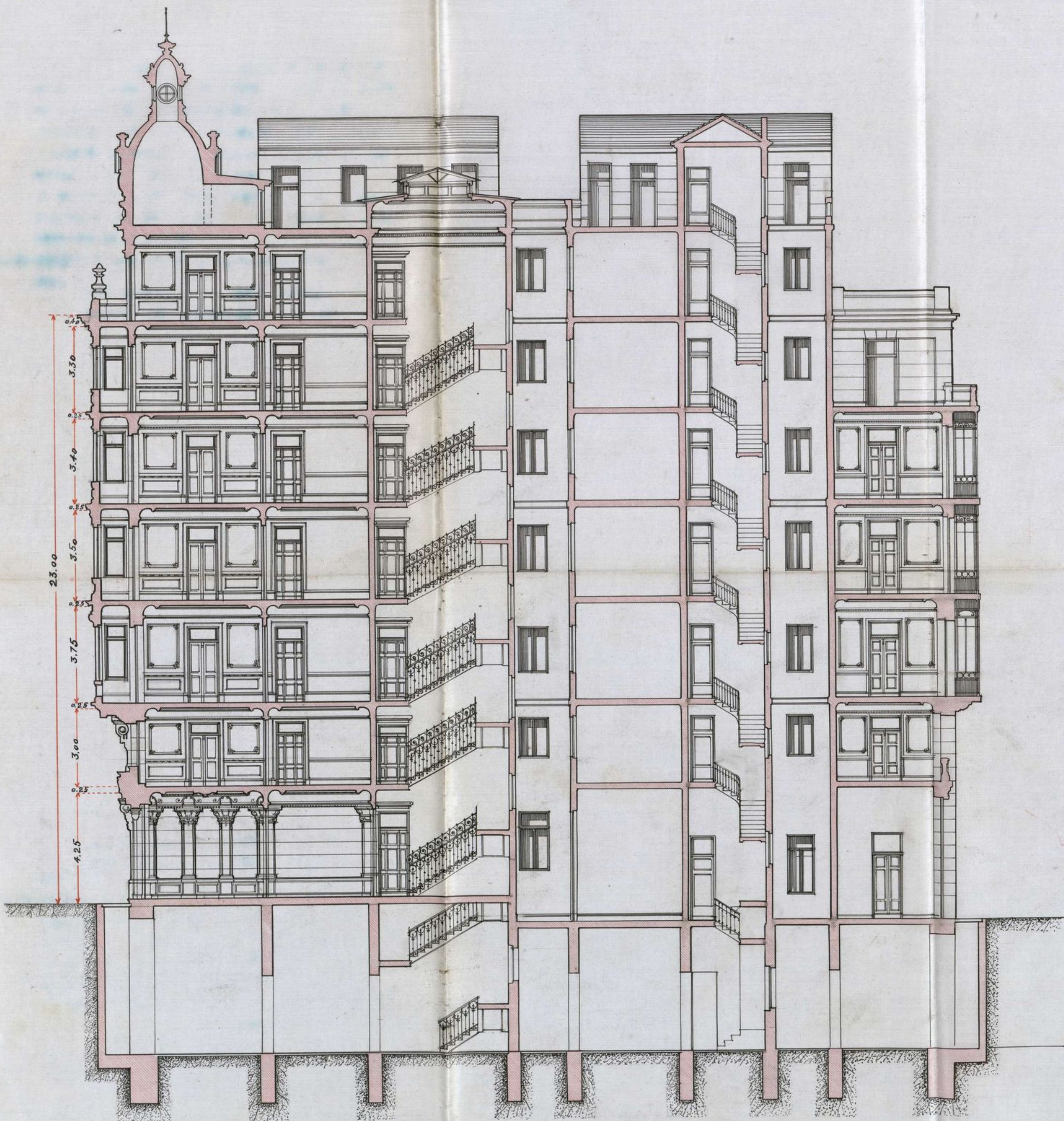
Sección por el eje.
