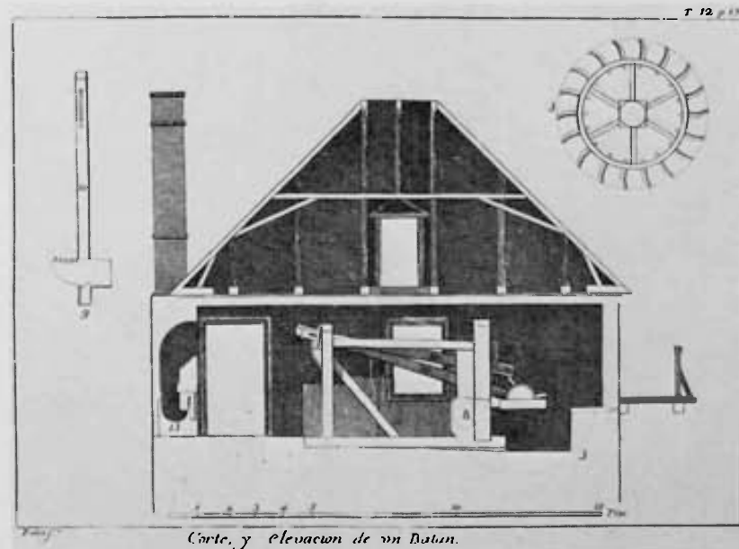
Corte, y elevacion de un Batán.
