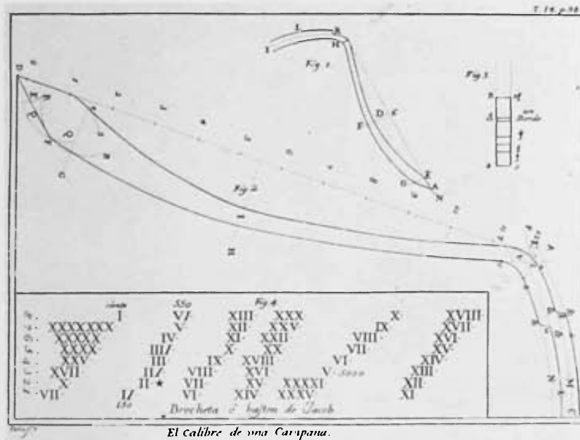
El Calibre de una Campana.
