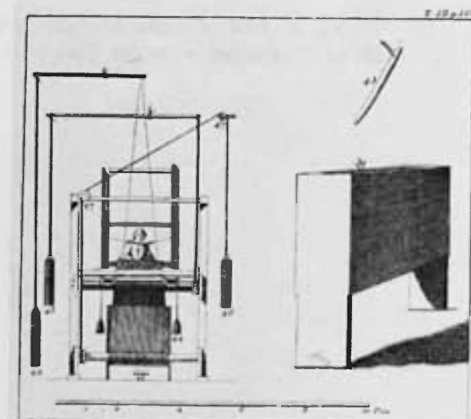
Telar para terciopelos visto de cara.
