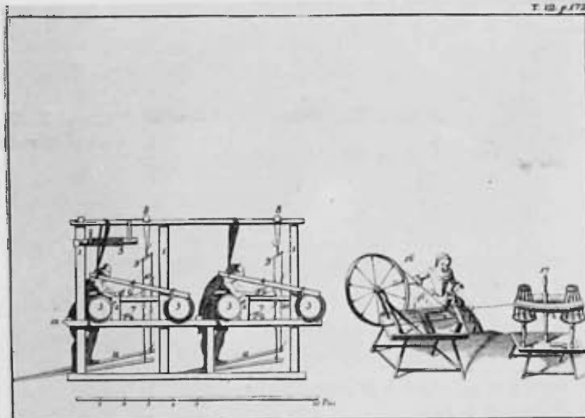
Lizos bajos horizontales.
