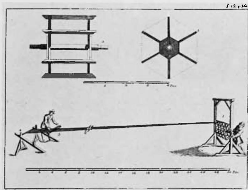
Modo de poner la Cadena en el Telar
