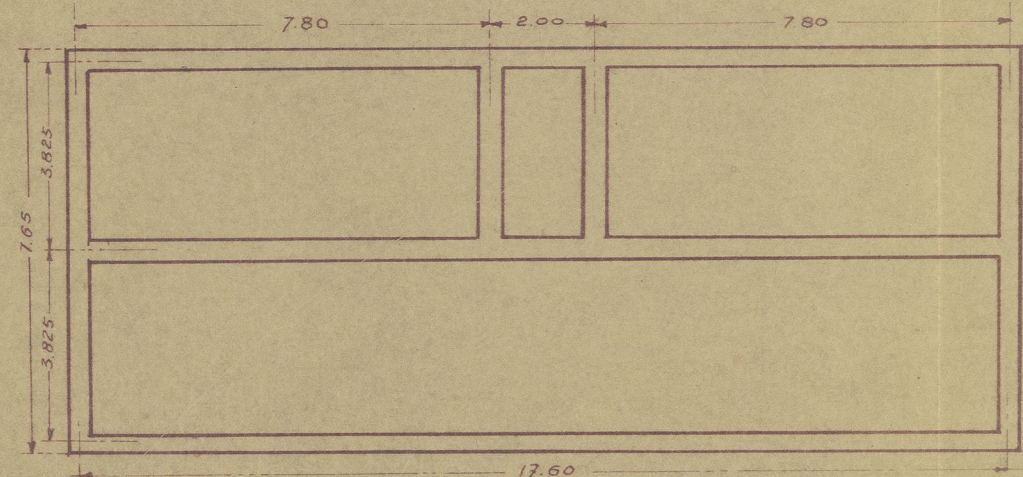
«Planta de cimientos.»
