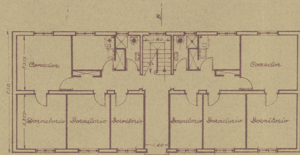
«Planta baja.»
