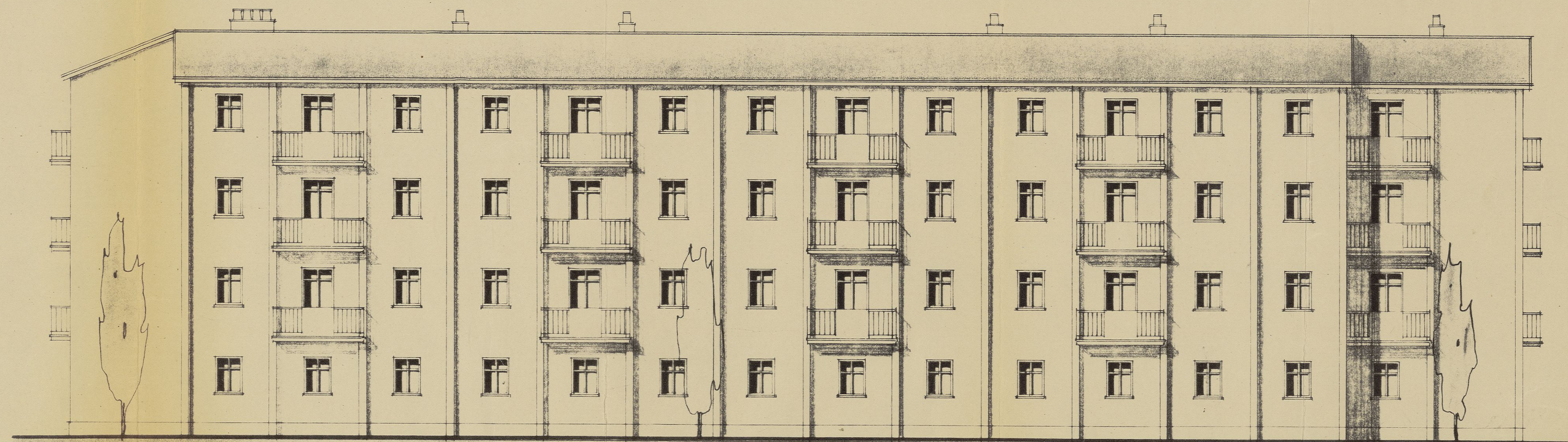
FACHADA POSTERIOR.
