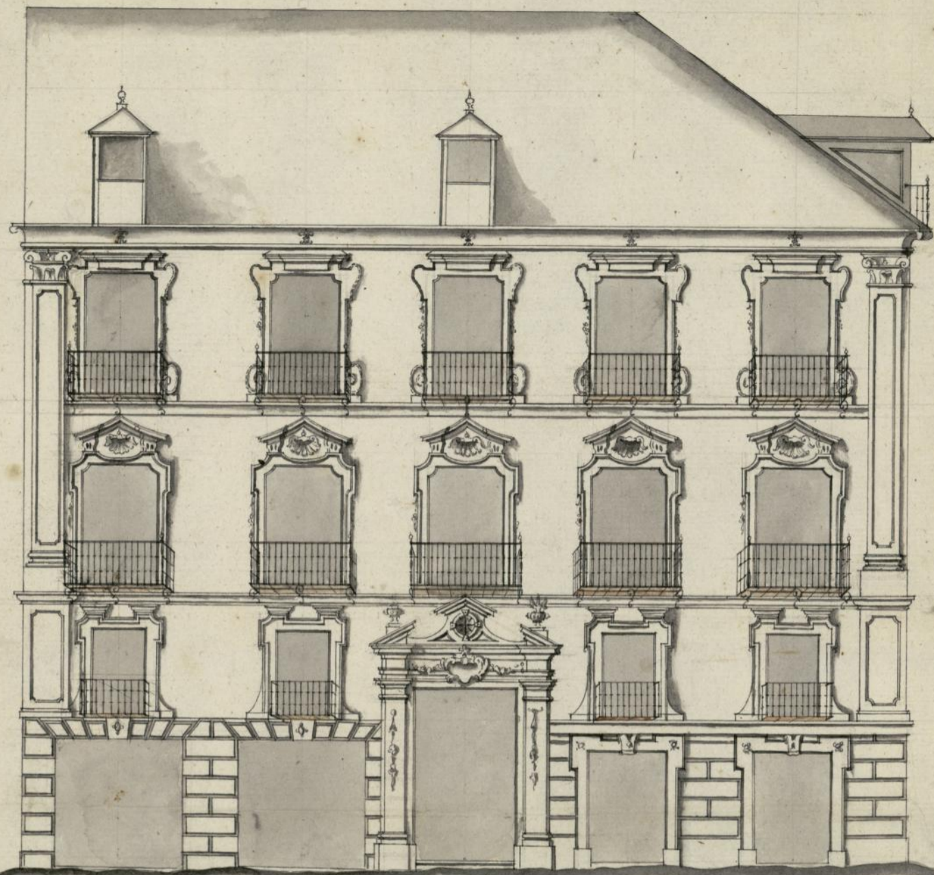
ALZADO DELA FACHADA QUE DA BISTA A LA PLAZUELA DE TRUJILLO;
