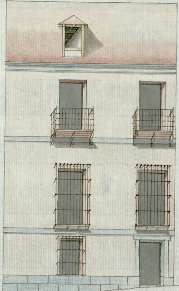
elevación de la fachada
