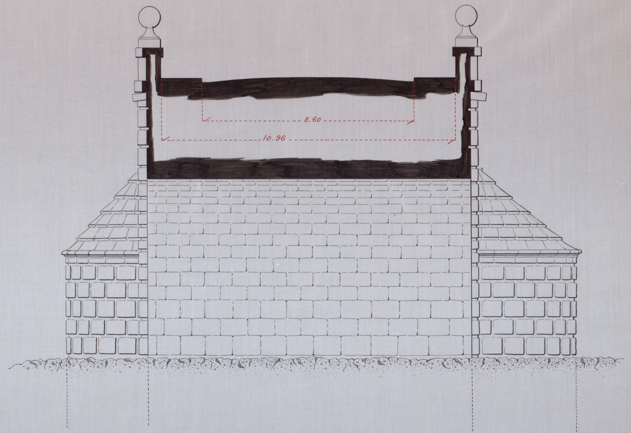
SECCION TRANSVERSAL
