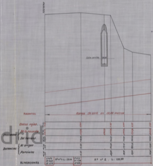
Perfil longitudinal
