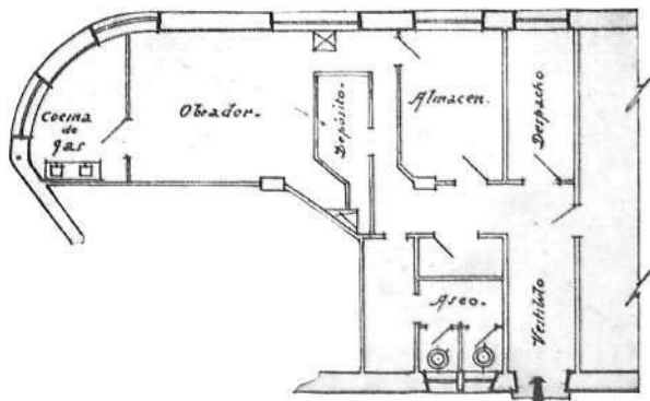
Planta de sótanos.
