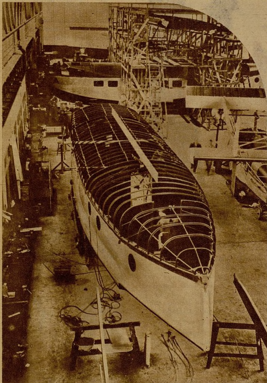
No es el esqueleto de una ballena. Se trata del casco de un avión anfíbio, destinado al servicio de correos de los Estados Unidos. Será el mayor del mundo y podrá desarrollar una velocidad de 129 millas (Foto Consorcio)
