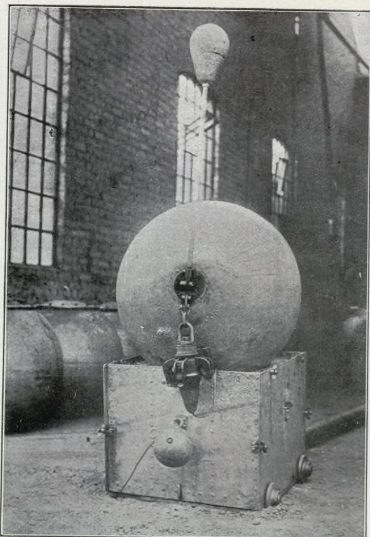
Nueva mina flotante de la marina inglesa (Fot. Branger)
