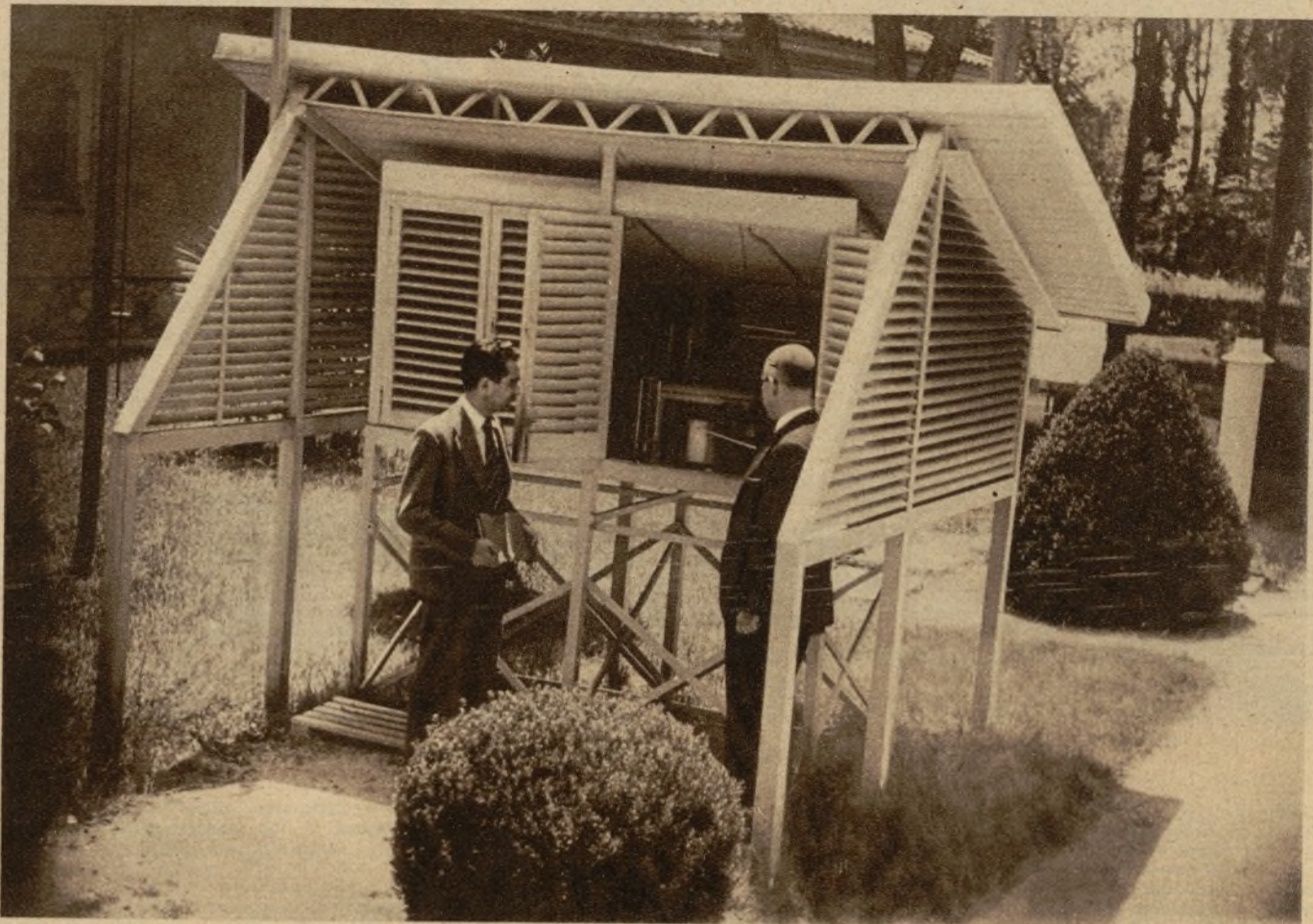
En esta caseta de madera se hallan encerrados los aparatos registradores de la temperatura del aire
