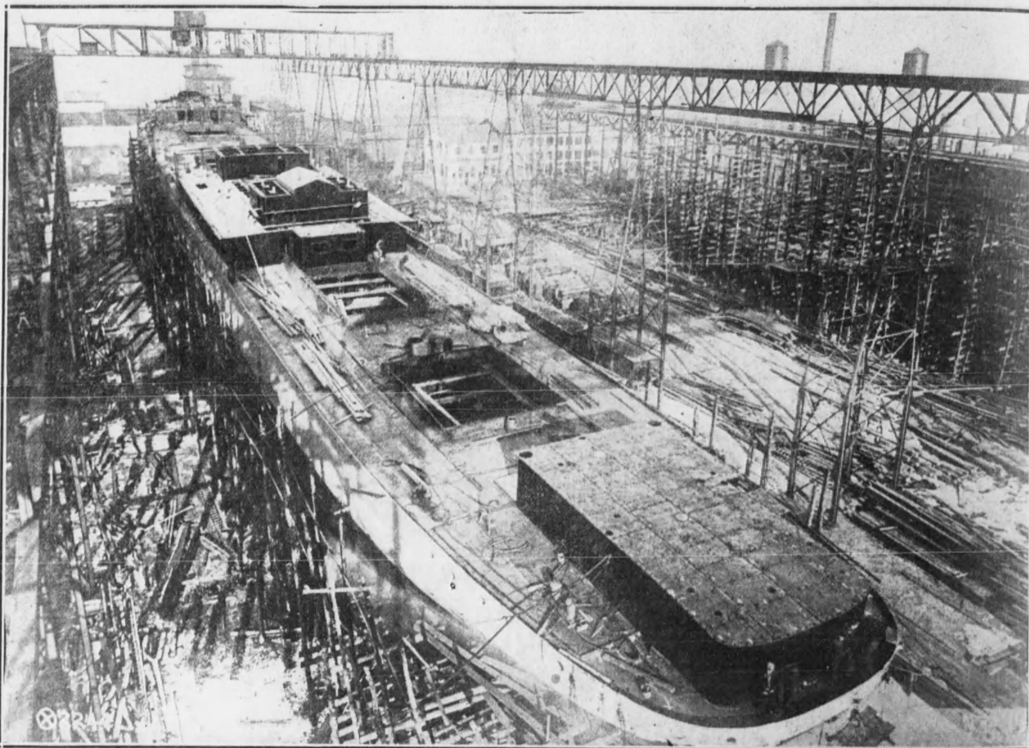
Uno de los inmensos navíos que en gran escala se están construyendo en los Estados Unidos, para el transporte de tropas y víveres a Europa
