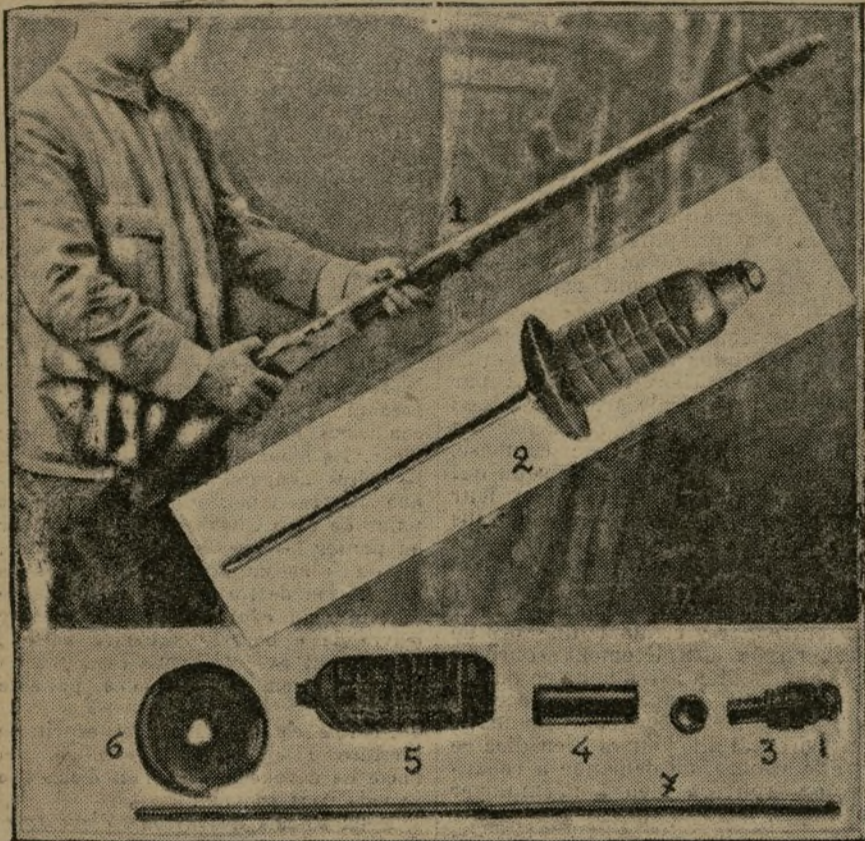
1. Le tir de la « queue de rat ». — 2. L'ensemble de l'engin. — 3. Bouchoir percuteur. — 4. Tube de cuivre interne. — 5. Grenade. — 6. Garde. — 7. Tringle.
