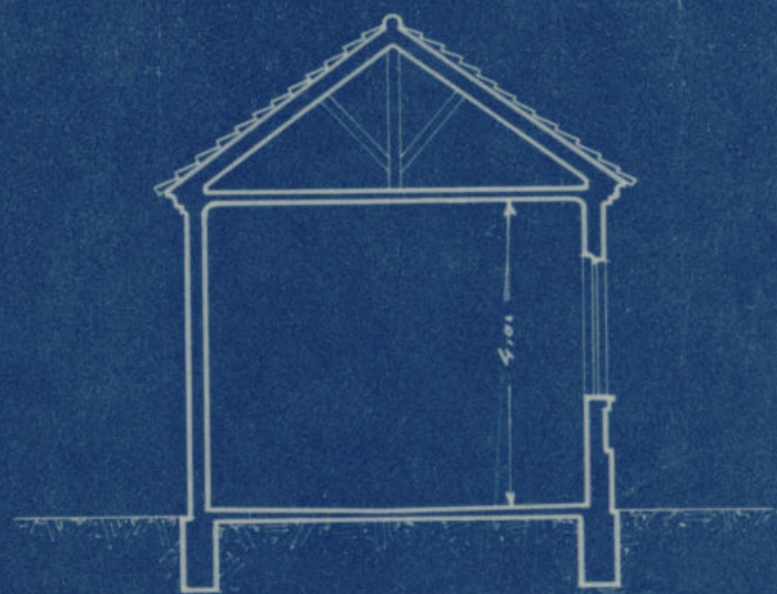
— SECCION —
