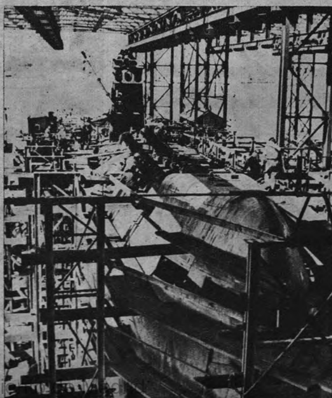
SUBMARINO ATOMICO.—En Connecticut, Estados Unidos, se dan los últimos toques al submarino atómico que será botado el 21 de enero próximo. Es el primero de su tipo, y podrá dar la vuelta al mundo a más de veinte nudos (Foto A. P.)
