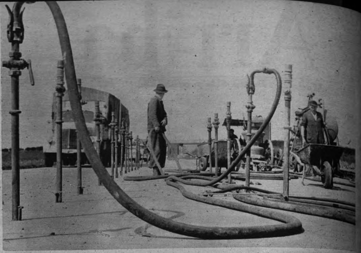
REMIENDOS A LA AUTOPISTA. —Los trabajos de reparación de la autopista alemana entre Hamburgo y Bremen se realizan con ayuda de un sistema de bombas que cubren los baches y refuerzan el pavimento de aquella famosa via terrestre de comunicación (Foto Cifra.)
