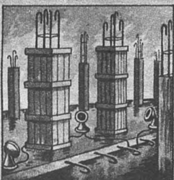
Para que las heladas no produzcan daño en el hormigón armado.
