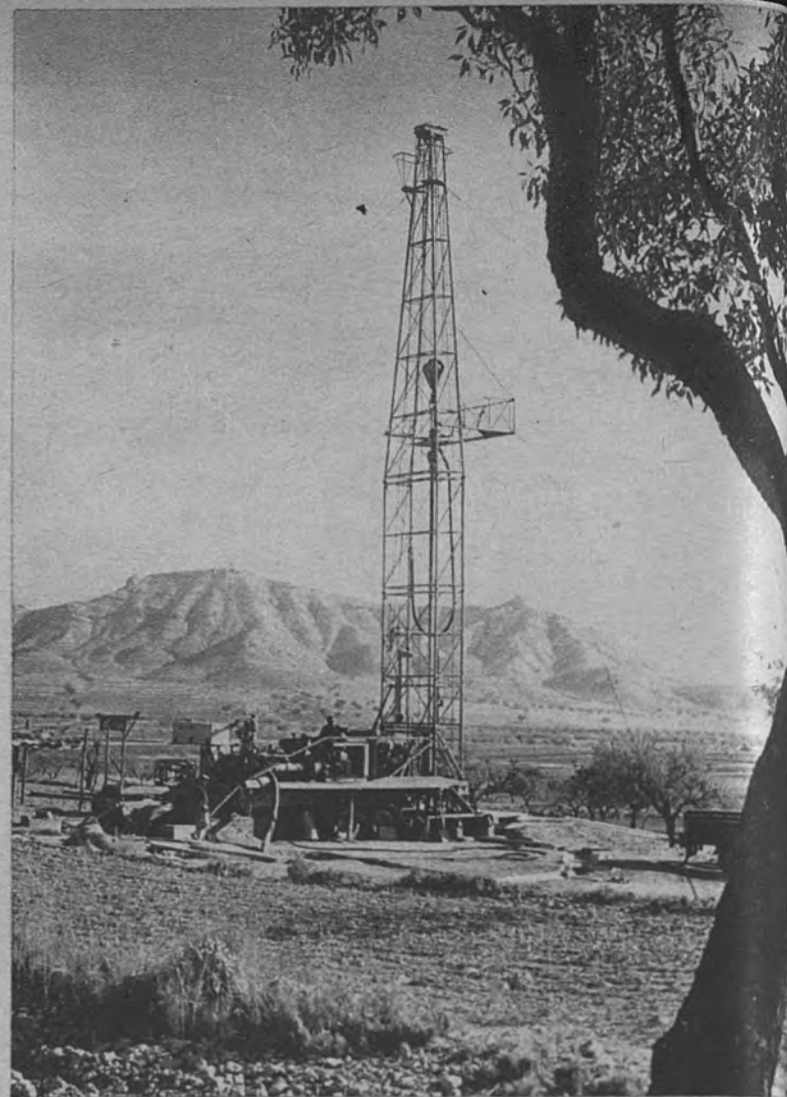
Equipo de sondeo «Failing 2.500», de los que utiliza el Instituto Nacional de Colonización para perforaciones profundas en el campo de Nijar
