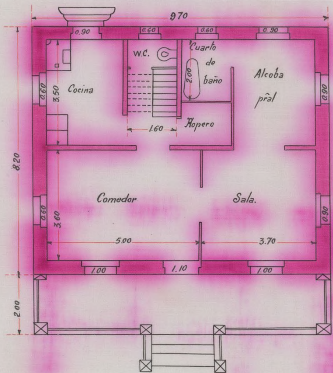
Planta Baja.
