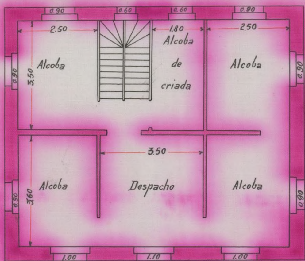
Planta pñal.
