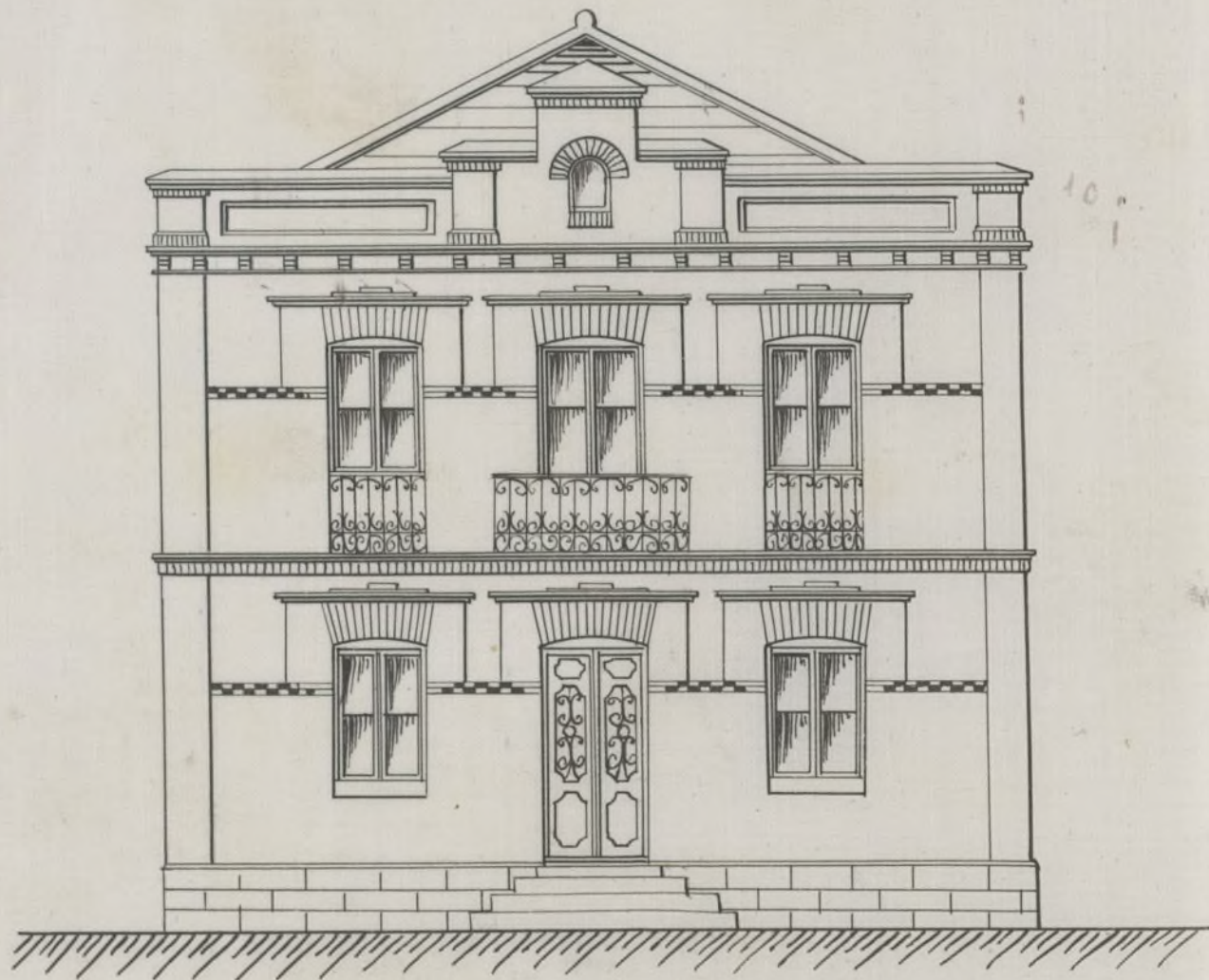
Alzado.
