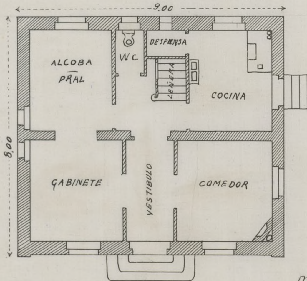
Planta.
