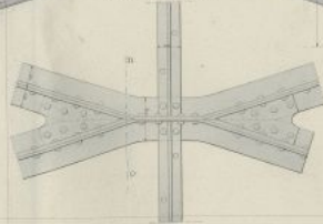
Croisement des fers.
