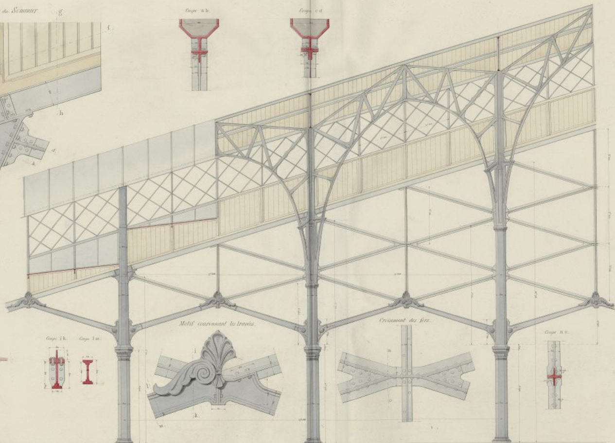
Assemblage de la Colonne et du Sommier.
