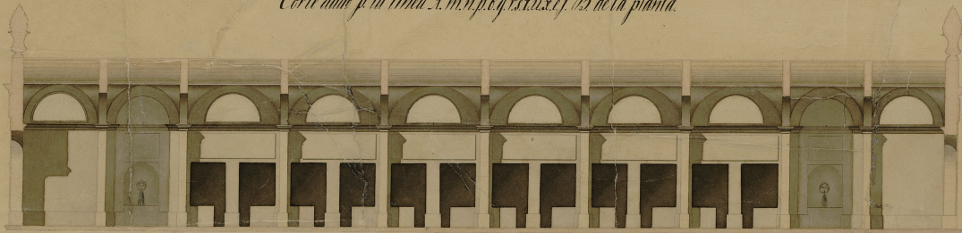
Corte dado p. o la linea C. D. de la planta.
