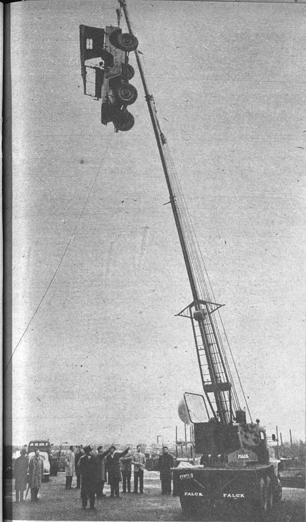
UNA GRUA POR TODO LO ALTO. —Una empresa danesa especializada en salvamentos ha encargado esta gigantesca grúa de gran potencia y fácil manejo que puede instalarse en la plataforma de un camión.—(Foto Fiel.)
