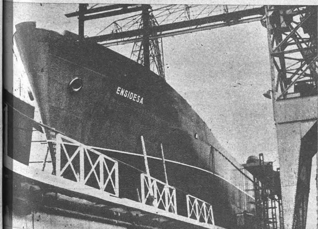
PREPARADO PARA ZARPAN. —En cuarenta y ocho días laborales ha sido montado el buque «Ensidesa» por los astilleros de Cádiz. Desplaza 6.400 toneladas y aquí aparece preparado para su botadura, que fue ayer. (Cifra.)
