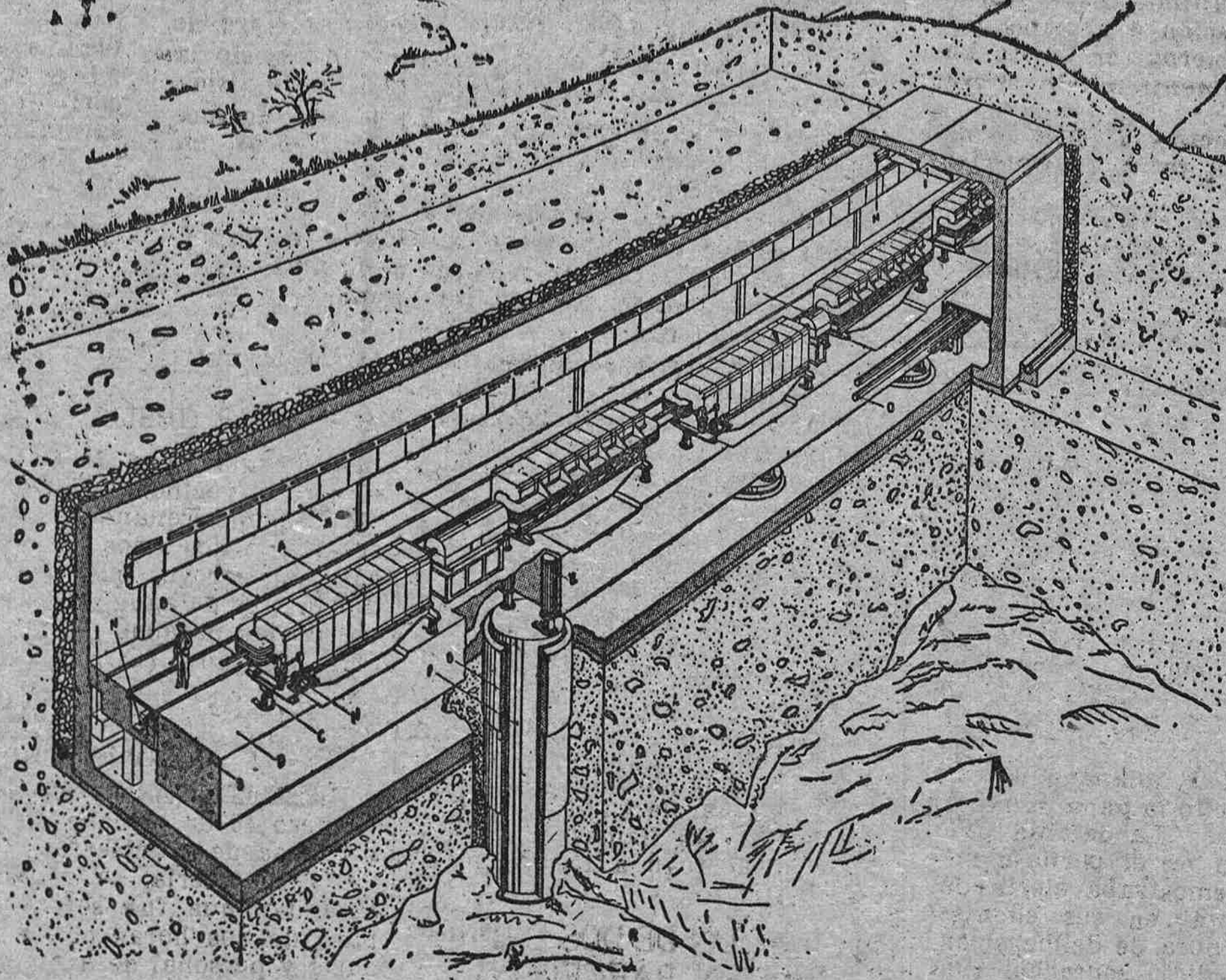
Corte y vista en perspectiva del edificio anular, de los cimientos, imanes, etc., del Centro Europeo de Investigaciones Nucleares, de Meyrin, cerca de Ginebra, recientemente inaugurado
