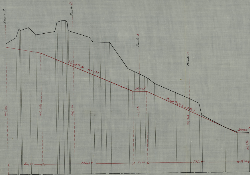
Perfil por el ege de la nueva calle que ha de sustituir al actual Paseo de Ronda de Recoletos
