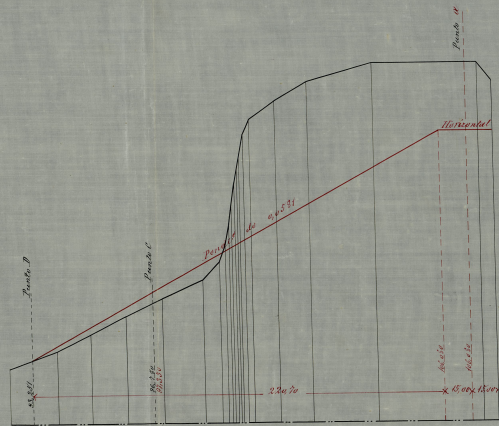
Perfil por el ege de la calle D C a Prolongacion de la Costanilla de S ta Feresa.
