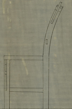
Seccion.
