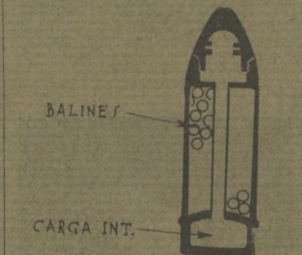
FIG. VII. BALINES. CARGA INT.
