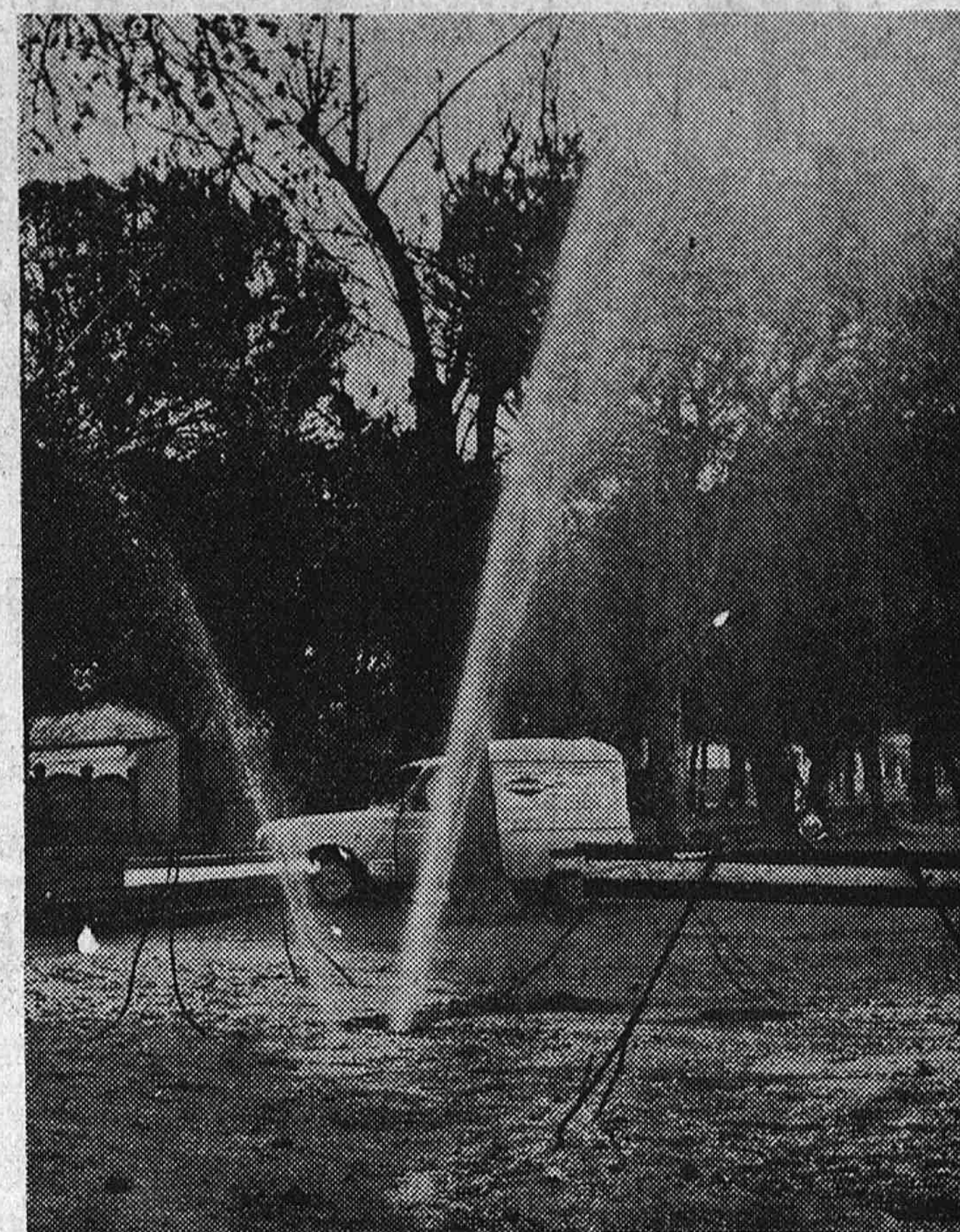
Para conocer el comportamiento de los componentes del subsuelo ante una vía de agua se construyó en el Instituto «Eduardo Torroja» una maqueta experimental (arriba), que reproduce un trozo de calle. El agua es inyectada por un tubo situado en el lado derecho. Como ilustra la imagen sobre estas líneas
