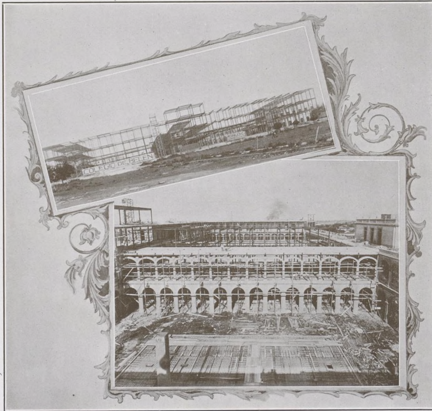
EL ARMAZON DE LA FACHADA EN 8 DE MAYO DEL 24. — LAS OBRAS Y CIERRE DEL ALGIBE EN 28 DE ENERO DEL MISMO AÑO.
