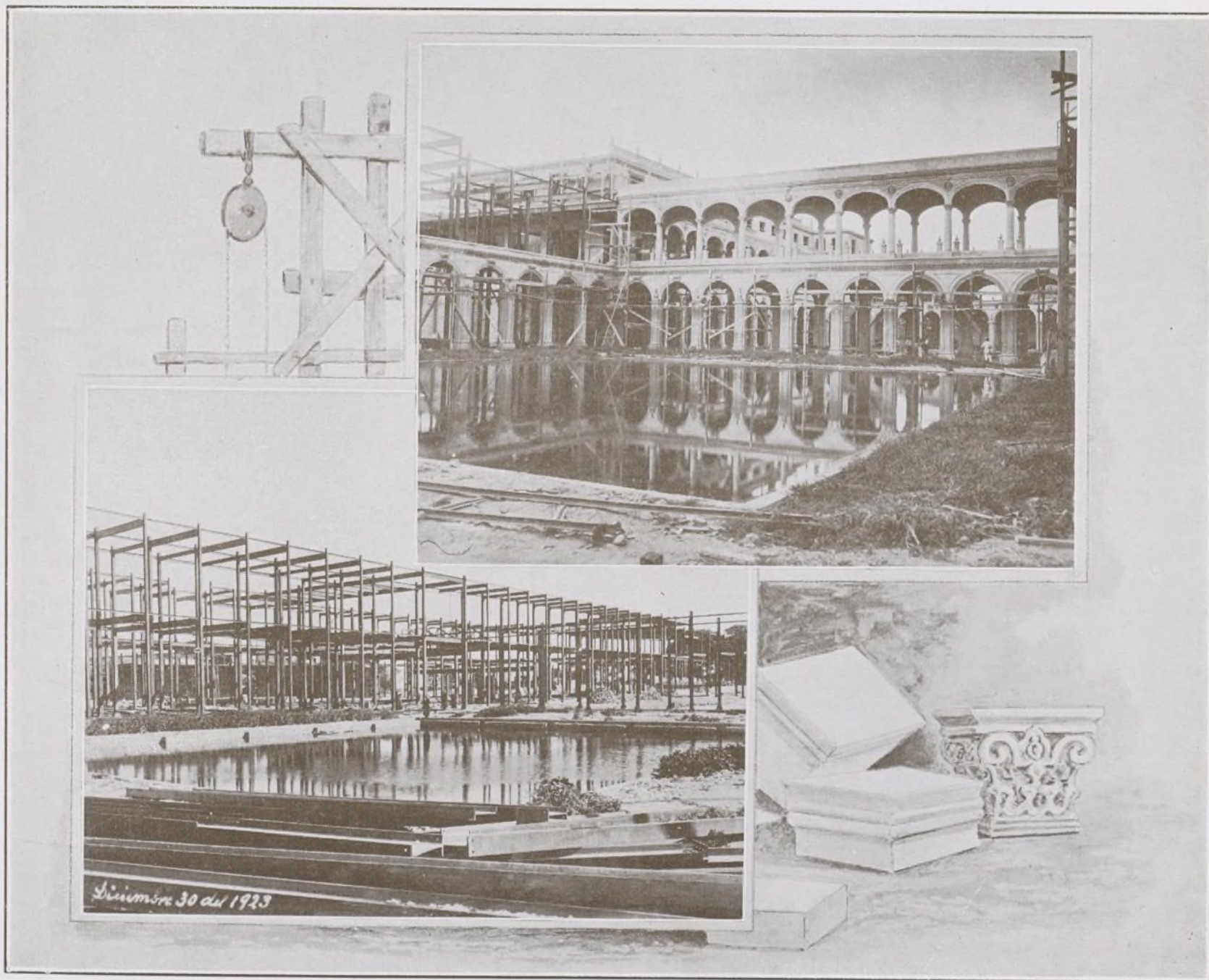
LAS OBRAS EN DICIEMBRE DE 1923 (EL ALJIBE DEL PATIO DE LA DERECHA, CUYAS AGUAS SE UTILIZARON PARA LA FABRICACION DEL COLEGIO.—LA PARTE MAS EDIFICADA ES DEL 15 DE JULIO DEL 24.)
