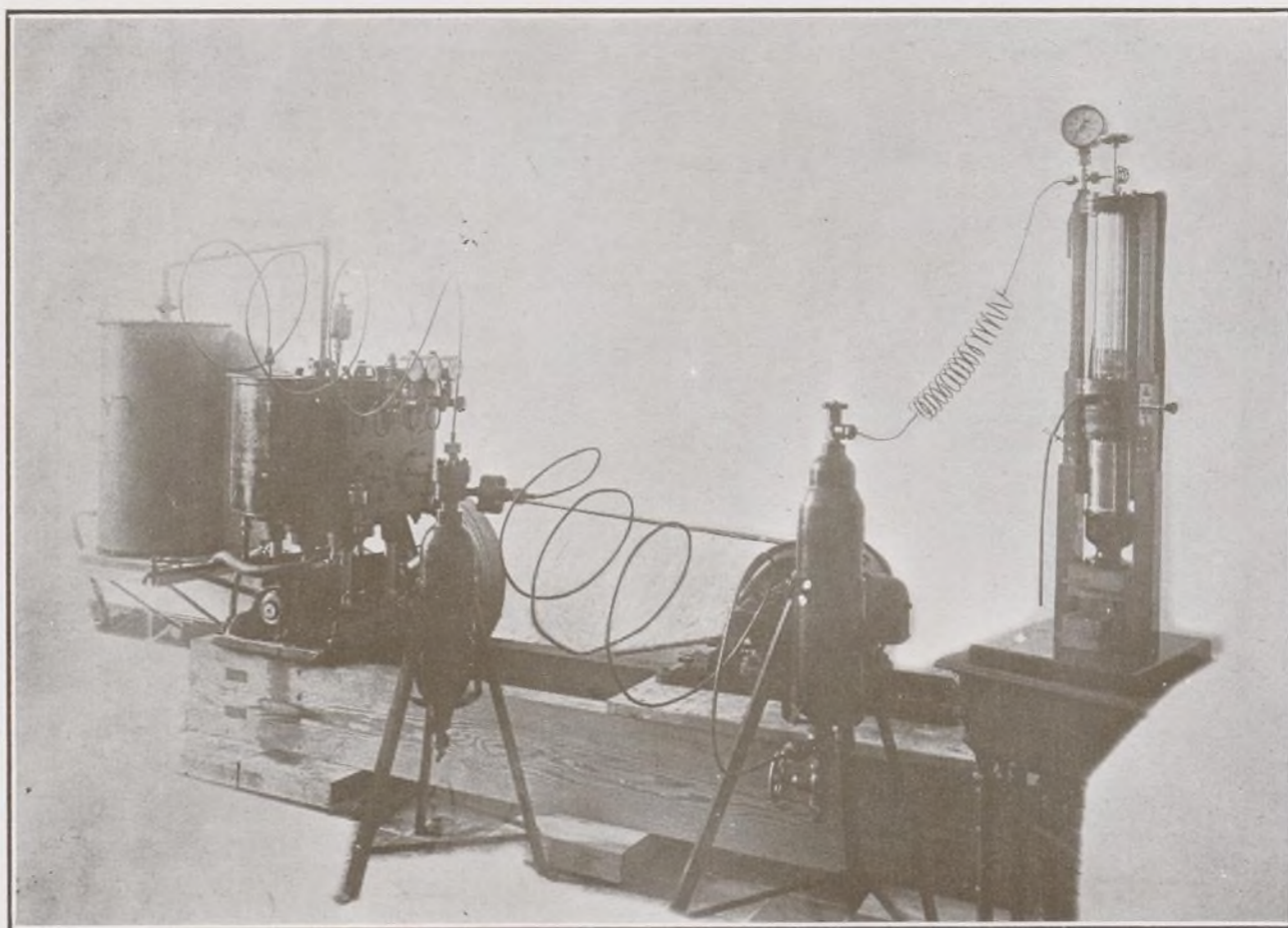
LA MAQUINA DE ELABORAR AIRE LIQUIDO.
